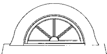
Type 90/55 B=90 cm - H=52 cm Bundhængt vinduesramme med udskyder
